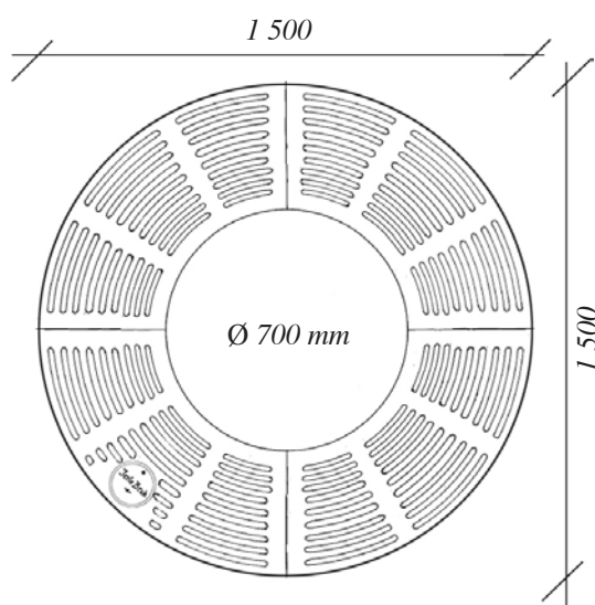
JB 602 Vikt: 96 kg
