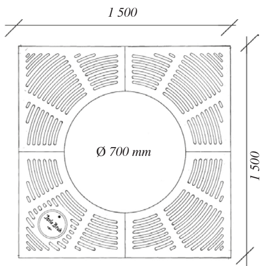
JB 601 Vikt: 128 kg
