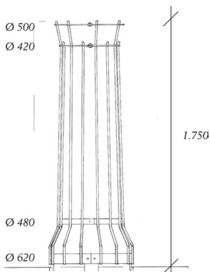
Stamskydd JB 451 Ø 600 Inklusive fästen
