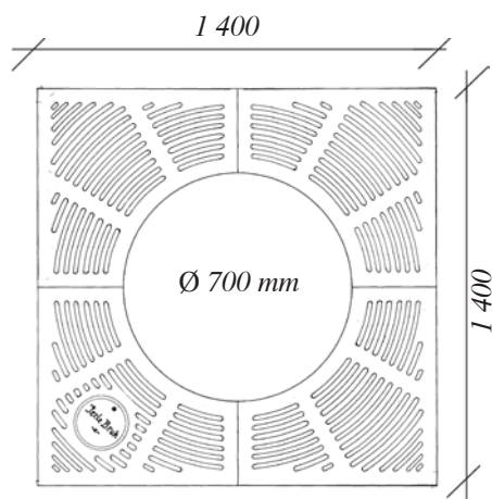
JB 603 Vikt: 100 kg
