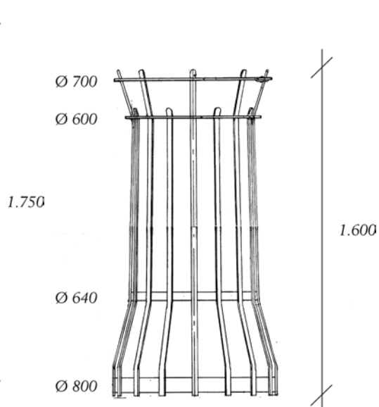
Stamskydd JB 453 Ø 800 Inklusive fästen
