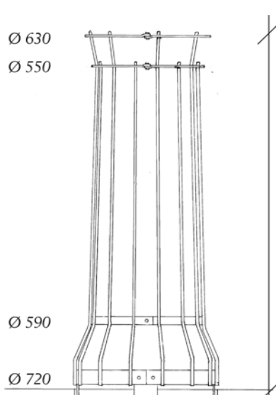
Stamskydd JB 452 Ø 700 Inklusive fästen
