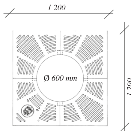
JB 604 Vikt: 72 kg
