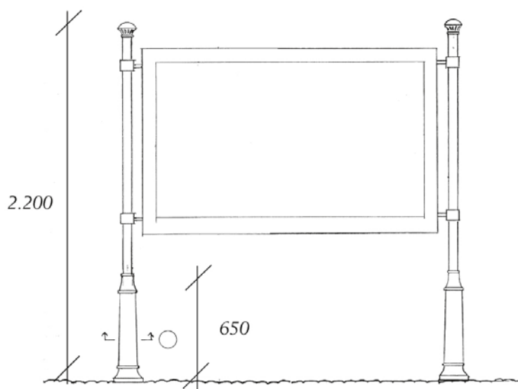
Stolpar till upplysningstavla JB 585
